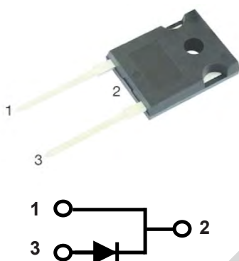
TO-247AC MURE6060APT-S
