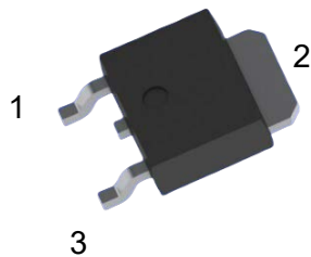
TO-252 MURE1660D
